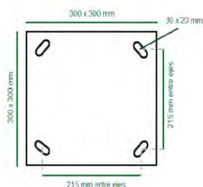
MEDIDAS PARA COLUMNAS DESDE 5 HASTA 6 METROS
